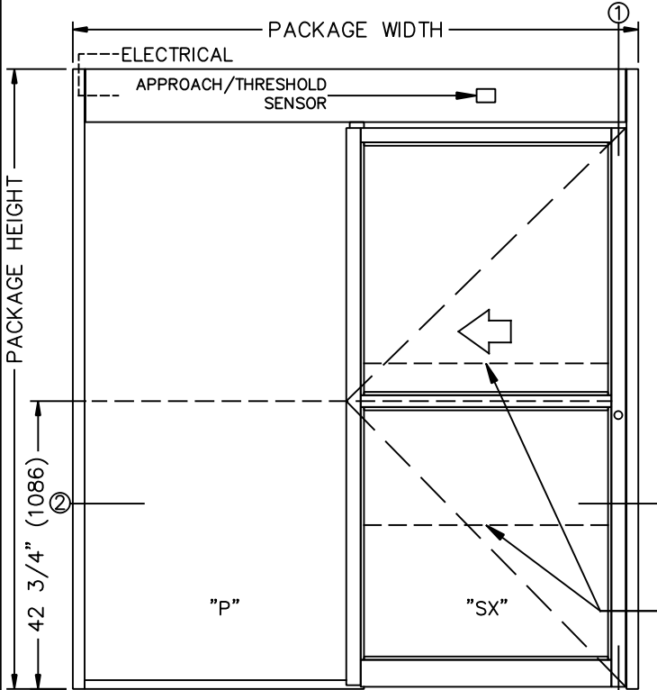
ELEVATION
