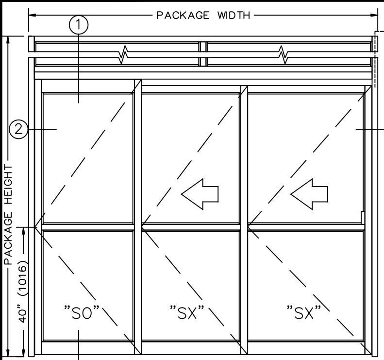
ELEVATION
